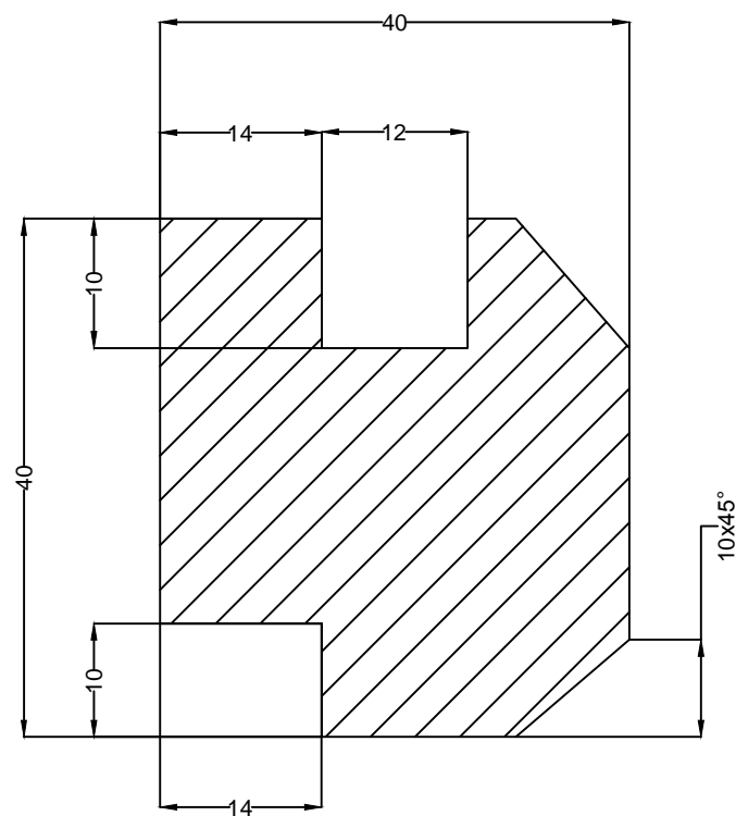
Е - Е
