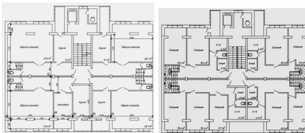
Рисунок.5 Планировочное решение двухуровневых квартир
